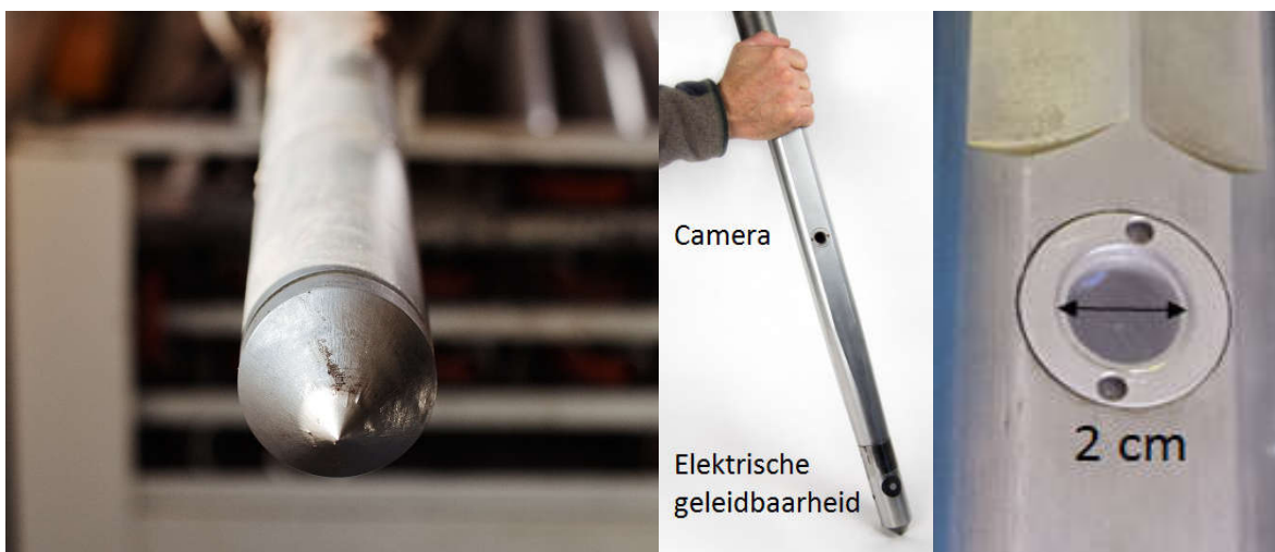
Elektrische CPT conus; camera- en elektrische geleidbaarheidsconus; grootte van het zijvenster voor de camera
