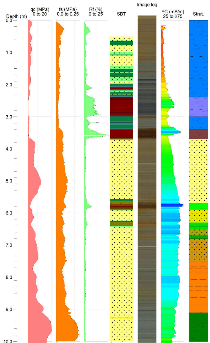
Camera-CPT te Prosperpolder Zuid v.l.n.r.: diepte, puntweerstand, plaatselijke wrijvingsgetal, wrijvingsgetal, Soil Behaviour Type (Koster 2016), camera image log, Elektrische Conductiviteit en geïnterpreteerde (litho-)stratigrafie.
